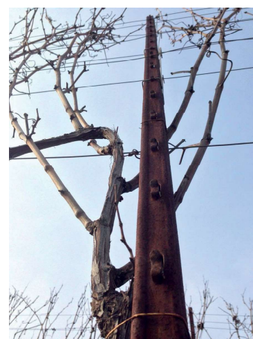
Piquets Intermédiaires de Vigne Cor- Ten avec Linguets
